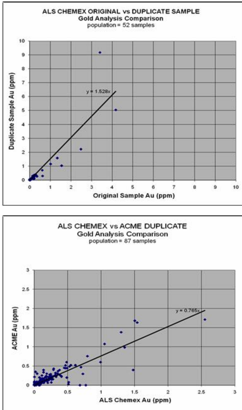
Figure 12.1: Original ALS Chemex versus ALS Chemex Duplicate Gold Analysis
