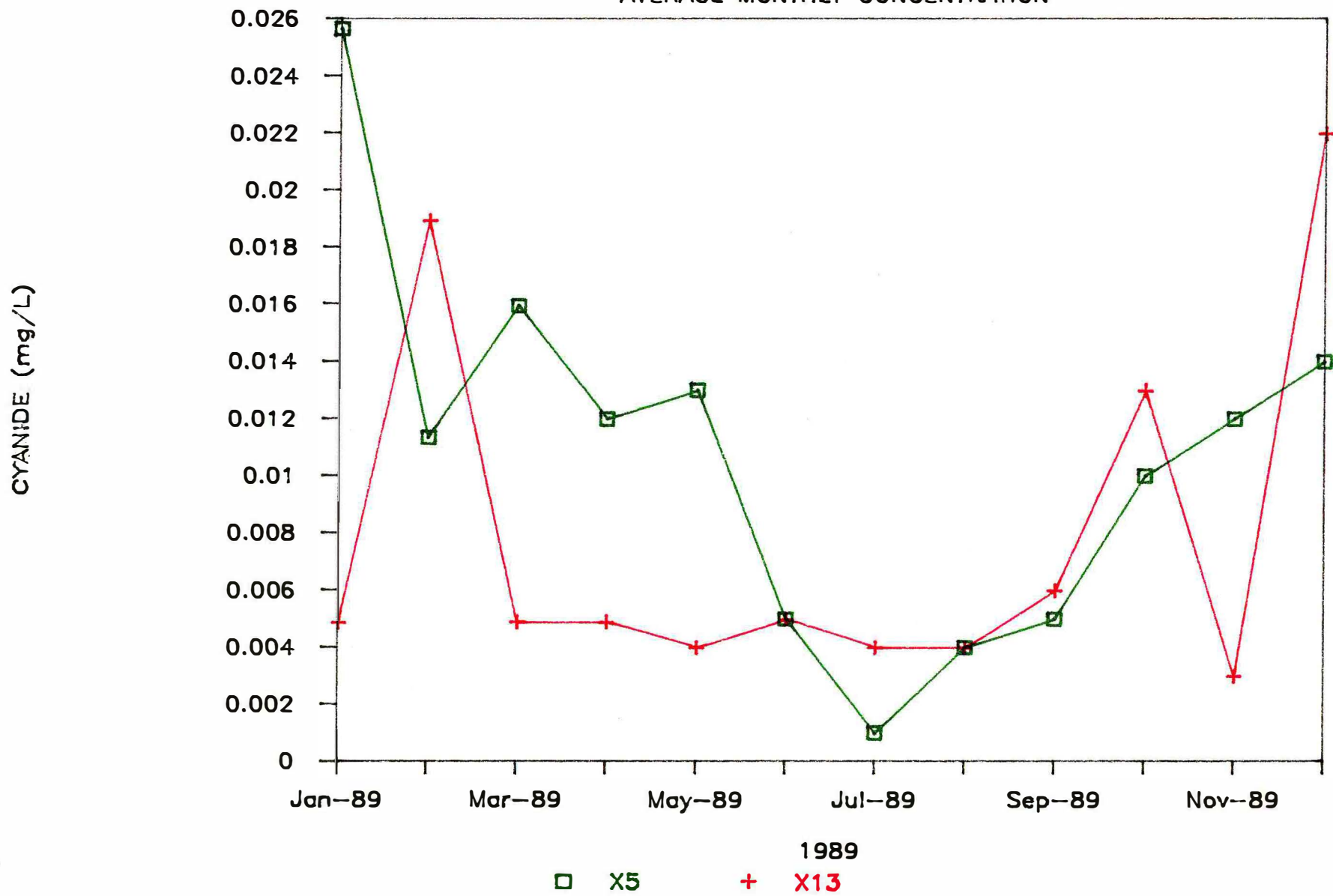
FIGURE 12 : CYANIDE (WAD)
